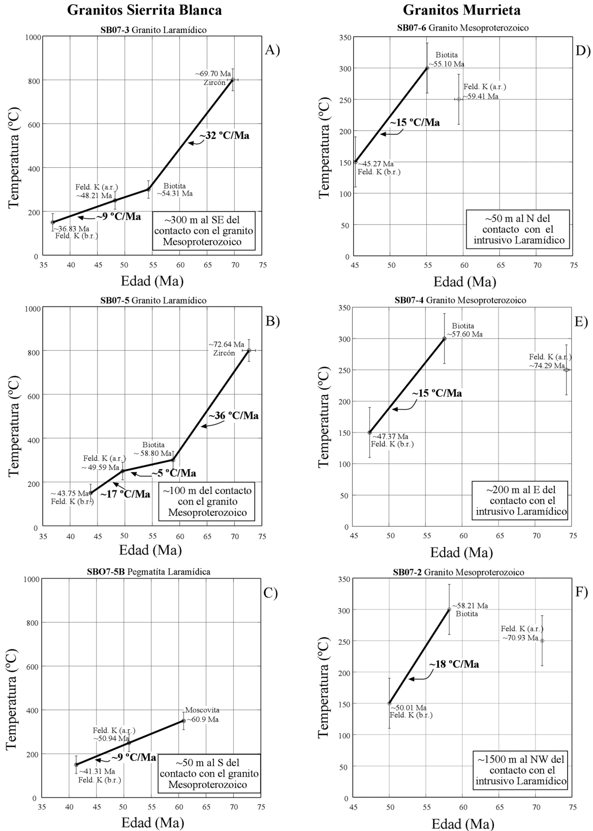
Figura 15. Curvas semi-cuantitativas de enfriamiento a partir de datos geocronológicos de U-Pb en zircones y 40 Ar/ 39 Ar en diferentes minerales para rocas graníticas de la Sierrita Blanca. A, B y C) Termocronología de los granitos laramídicos Sierrita Blanca, incluyendo una pegmatita tardimagmática de aproximadamente la misma edad (~61 Ma, moscovita). D, E y F) Termocronología de granitos mesoproterozoicos Murrieta. En cada uno de los gráficos se indica la velocidad de enfriamiento entre varios pares minerales (ej., biotita-feldespatos), y a que distancia fueron recolectadas las muestras con respecto al contacto intrusivo-encajonante.
